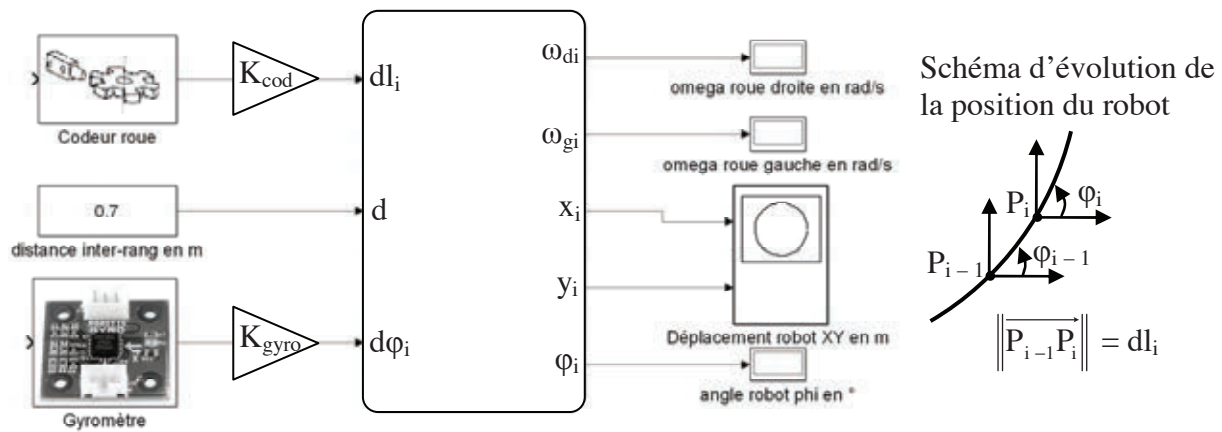
Figure 18 - Entrées/sorties carte Arduino Méga.
