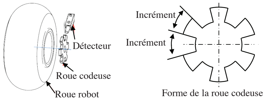
Figure 19 - Codeur incrémental équipant les roues.
