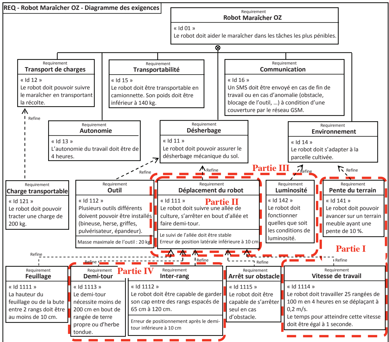
Figure 2 - Diagramme partiel des exigences.
