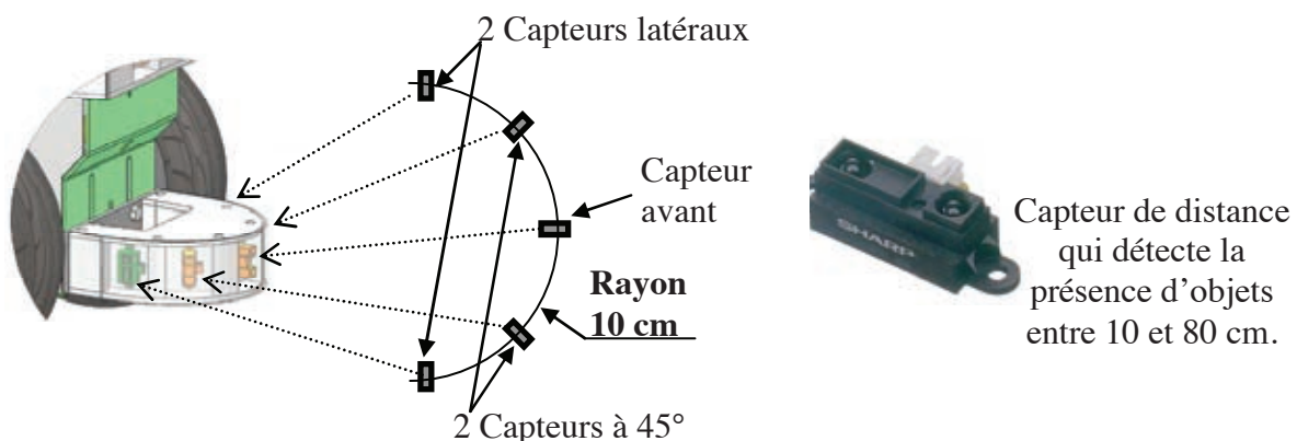
Figure 9 - Localisation des capteurs de distance.
