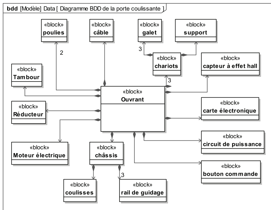
Figure 9 – Diagramme BDD de la porte coulissante
