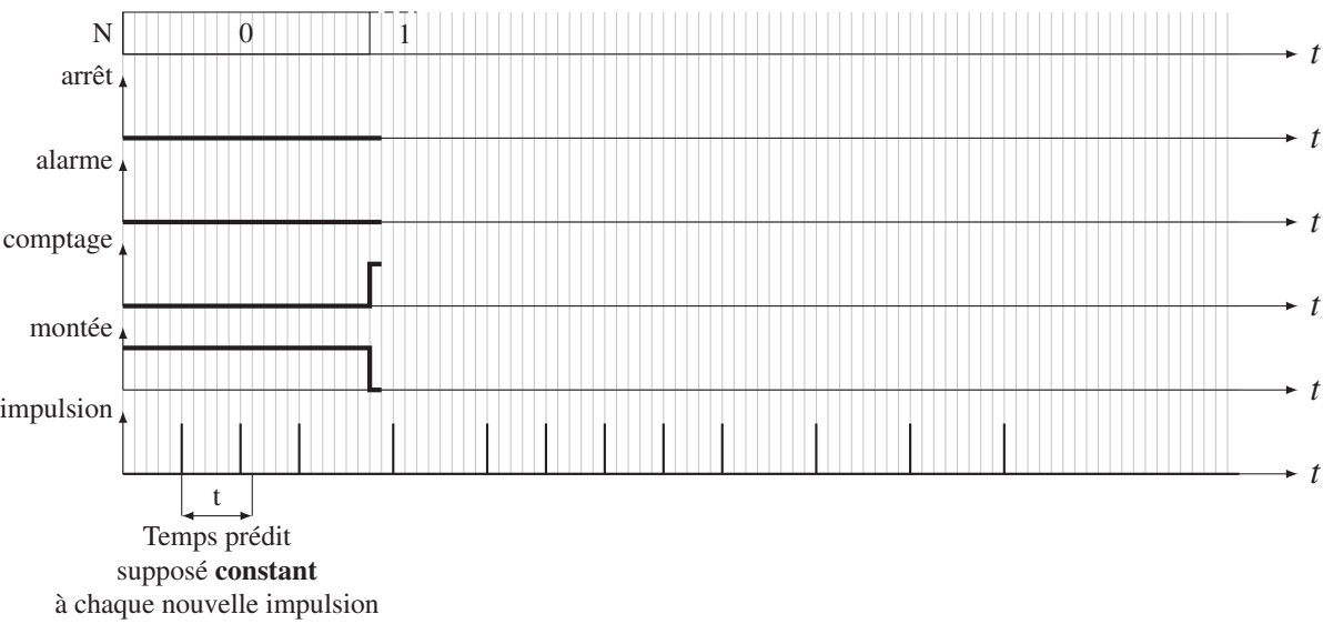
DR 4 – Chronogramme à compléter
