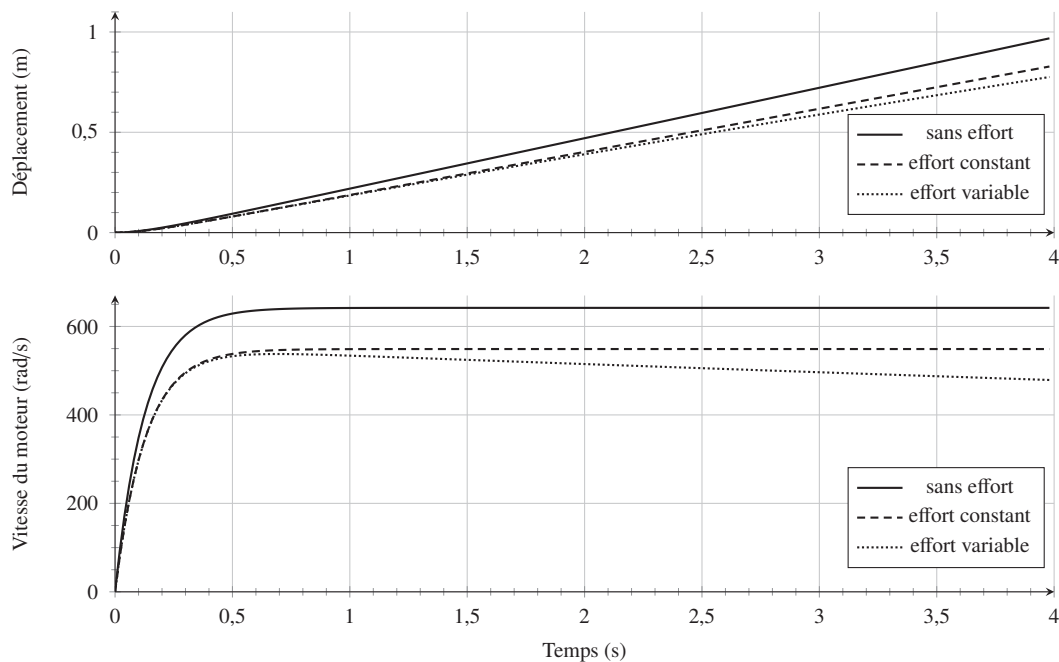
Figure 11 – Courbes de la position de la vitre et de la vitesse de rotation du moteur
