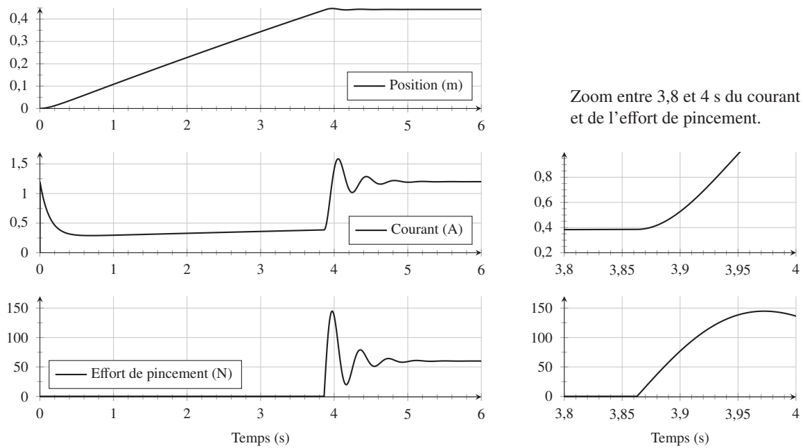
Figure 12 – Courbes de position de la vitre, d'intensité moteur et d'effort de pincement
