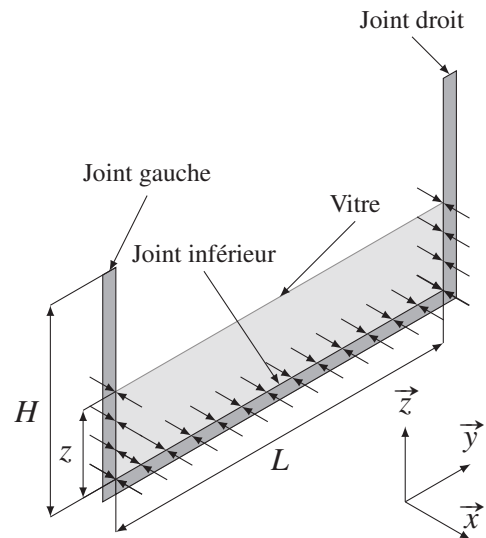
Figure 10 – Paramétrage et représentation des efforts normaux uniquement
