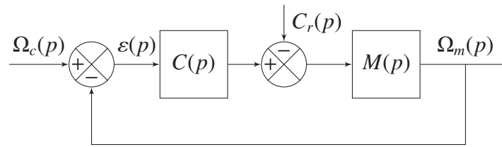
Figure 16 – Schéma-blocs équivalent de l'asservissement de vitesse du moteur
