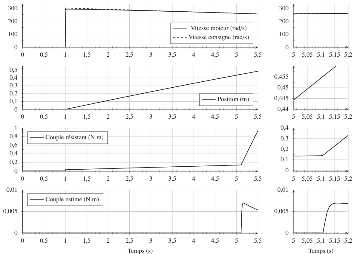
Figure 17 – Courbes de vitesse et de position, courbes du couple résistant et du couple généré par l'obstacle estimé (zoom entre 5 et 5,2 s à droite)
