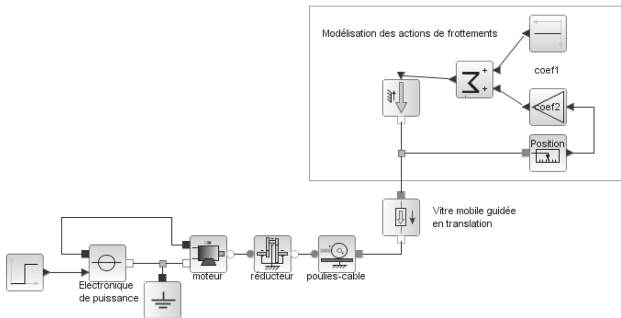
DR 3 – Schéma-blocs à compléter
