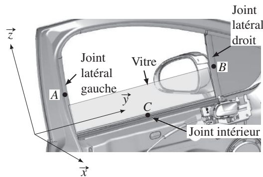
Figure 6 – Implantation et repérage des joints
