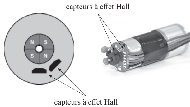
Figure 13 – Principe du capteur à effet Hall
