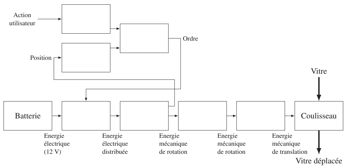
DR 1 – Chaînes fonctionnelles du lève-vitre électrique
