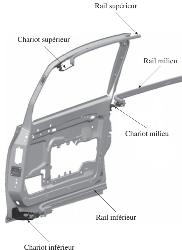
Figure 8 – Description du système de guidage de la porte coulissante électrique
