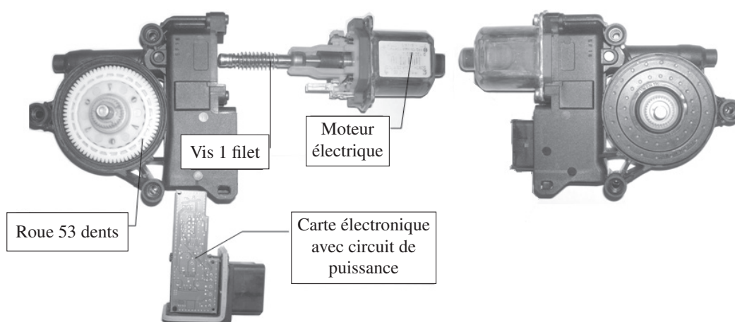
Figure 19 – Eclaté du moto-réducteur
