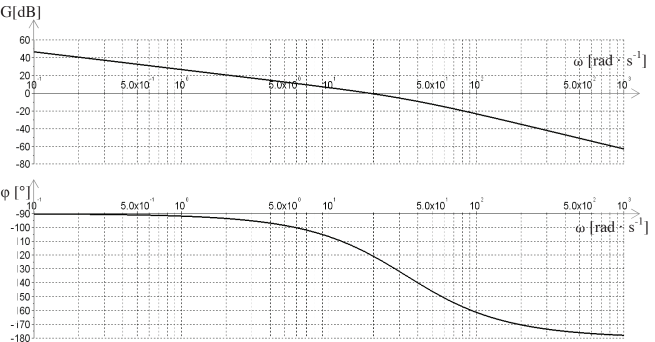
Diagramme de Bode de H_{bo}(p) pour K_p = 1
