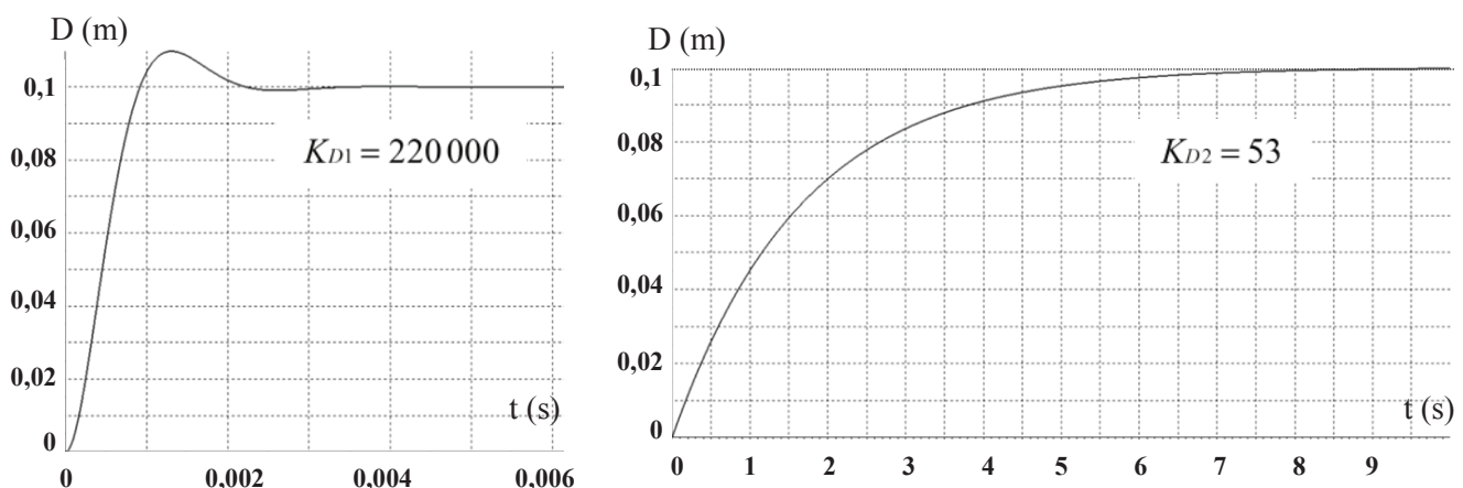
Figure 13 – Réponses indicielles du système asservi
