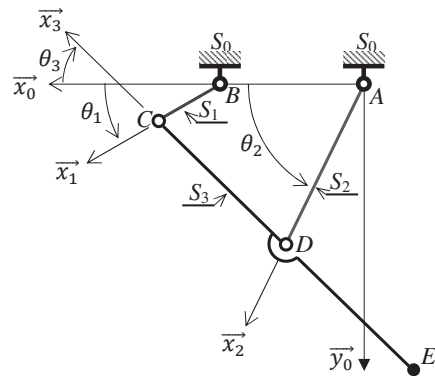
Figure 5 – Modélisation cinématique
