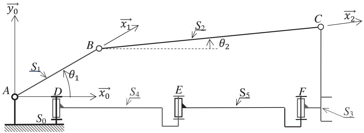
Figure 13 – Modélisation cinématique
