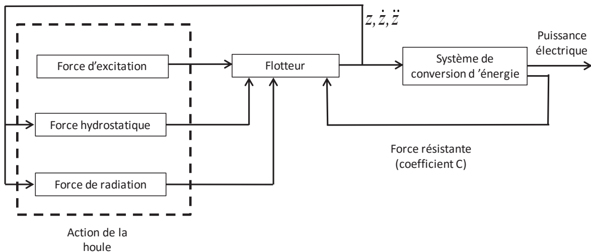
Figure 8 - Modèle multiphysique
