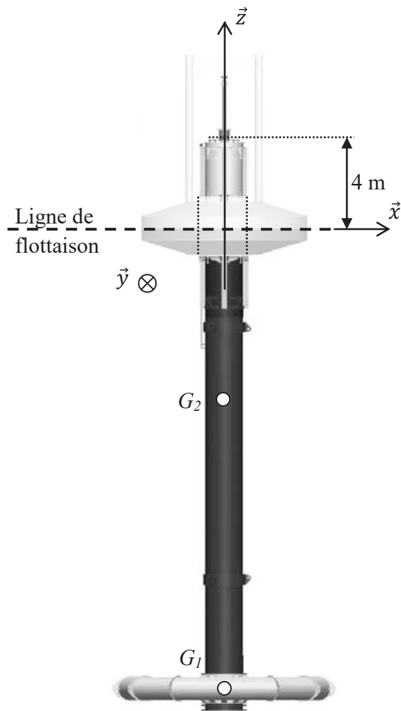
Figure 6 - Bouée en configuration verticale
