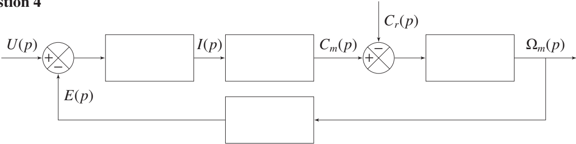
DR1 – Schéma-bloc des moteurs de propulsion
