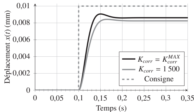
Figure 18 – Réponses temporelles x(t) du système réel perturbé à un échelon en déplacement de valeur finale X_c = 10 mm, pour une correction proportionnelle K_{corr} = 1\,500 et pour K = K_{corr}^{MAX}
