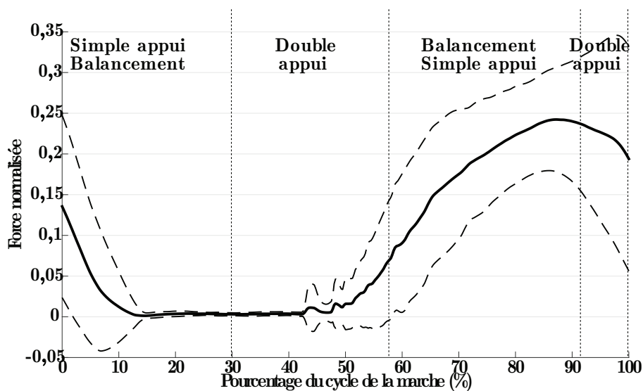
Figure 7 – Efforts normaux générés par la canne durant un cycle de marche assistée à allure moyenne, V = 0,22 m/s
