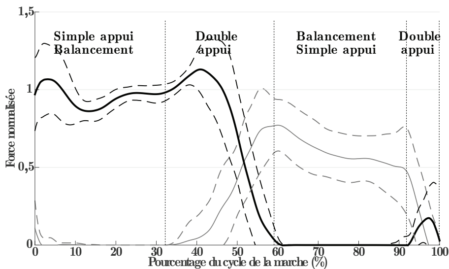
Figure 6 – Efforts normaux générés par les jambes durant un cycle de marche assistée à allure moyenne, V = 0,22 m/s
