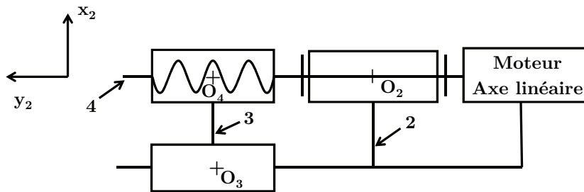
Figure 15 – Modélisation cinématique de l'axe linéaire
