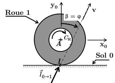
Figure 14 – Bilan partiel des actions mécaniques exercées sur la roue 1
