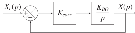
Figure 16 – Schéma-bloc simplifié du système non perturbé avec C(p) = K_{corr}
