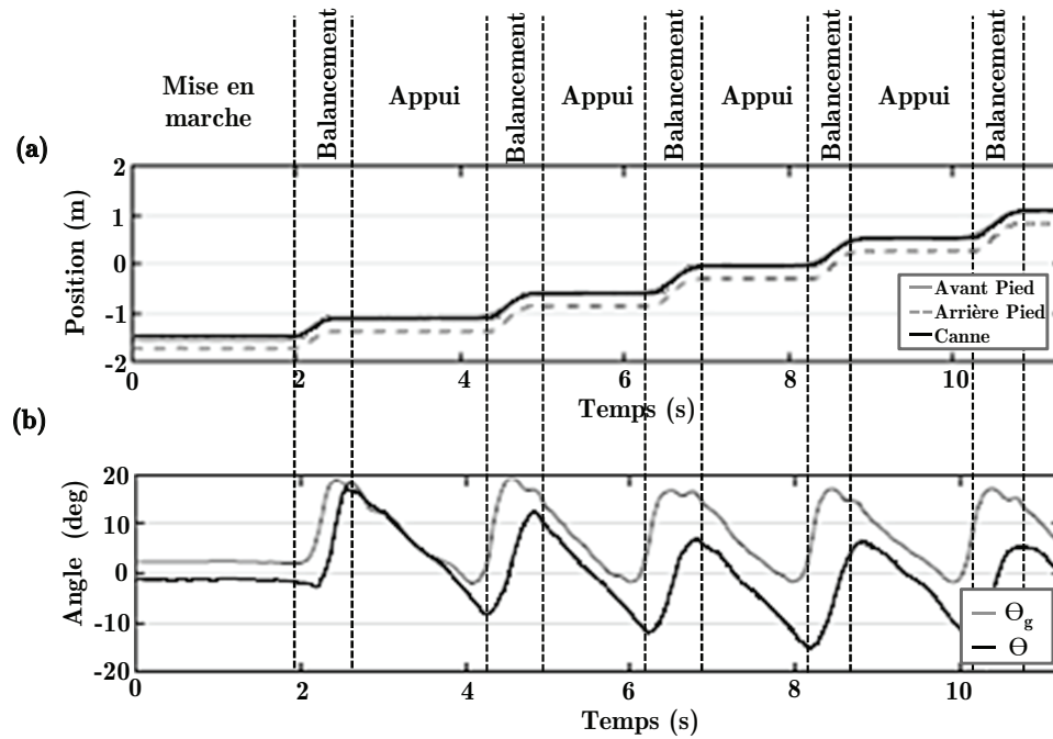
Figure 23 – V = 0,29 m/s, allure rapide – (a) : suivi du pied de la jambe gauche par la canne observé au niveau du sol – (b) : suivi de l'orientation de la cuisse gauche (angle \theta_g ) par la canne (angle \theta )
