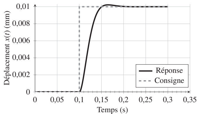
Figure 17 – Évolution de la réponse temporelle x(t) du système réel non perturbé à un échelon de valeur X_c = 10 mm, pour K_{corr} = 1\,500
