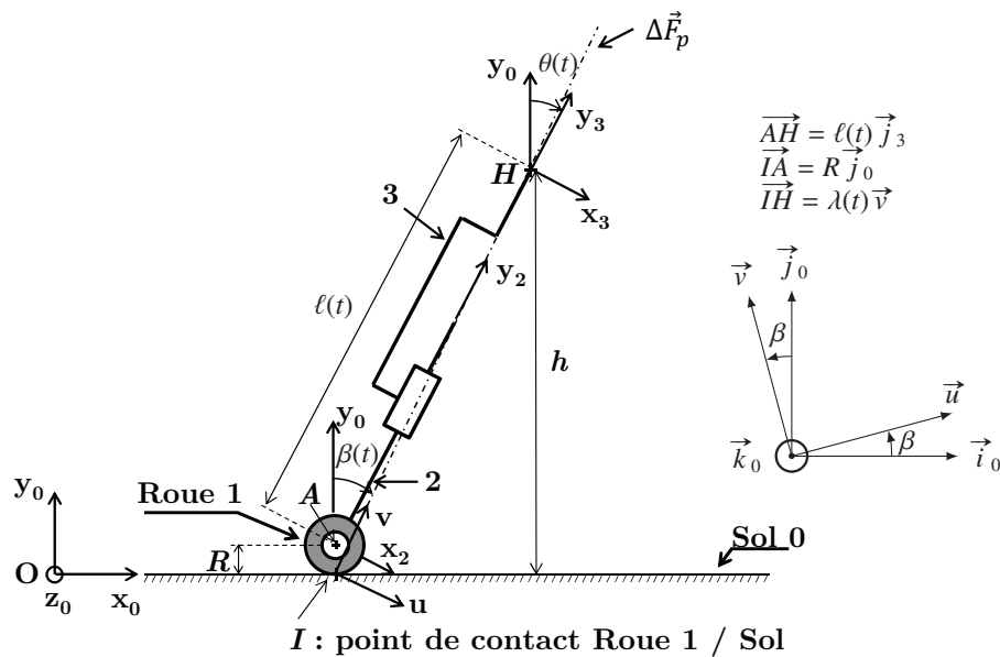
Figure 13 – Modélisation et paramétrage du prototype de canne robotisée
