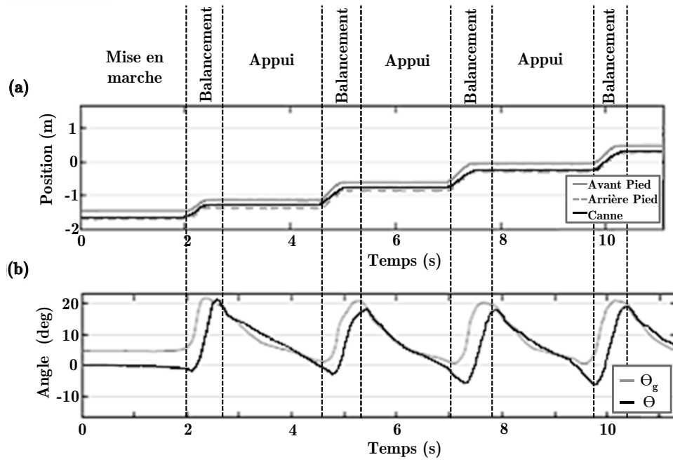
Figure 22 – V = 0,22 m/s, allure normale – (a) : suivi du pied de la jambe gauche par la canne observé au niveau du sol – (b) : suivi de l'orientation de la cuisse gauche (angle \theta_g ) par la canne (angle \theta )
