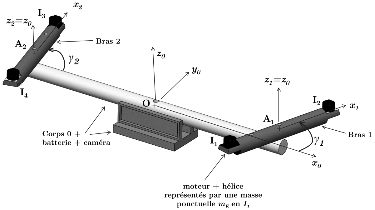
Figure 6 - Figure simplifiée de la géométrie du drone
