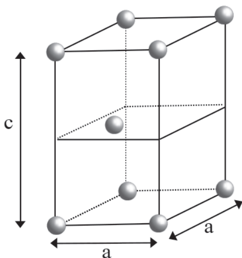
FIGURE 6 – Maille du titane ( \alpha )
